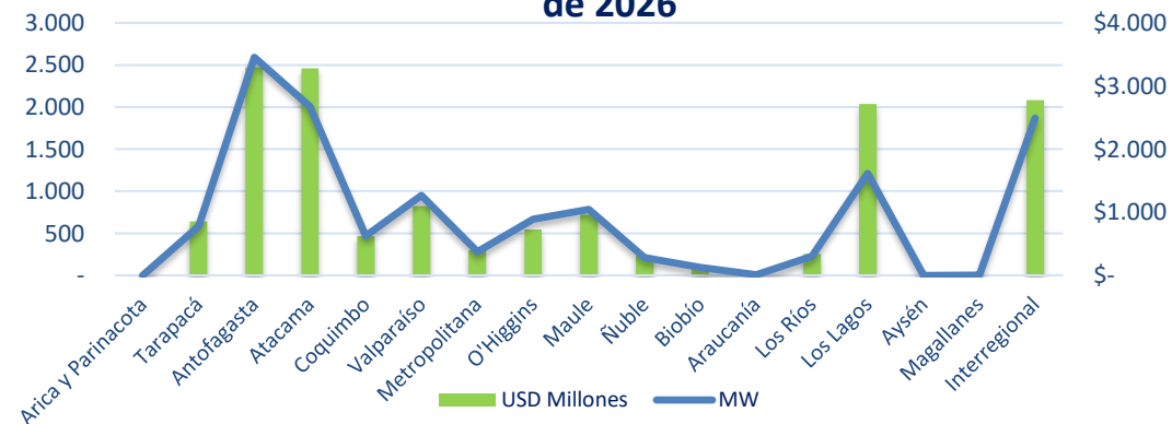
Inversión en USD millones y capacidad en MW de centrales de generación en calificación al 31 de agosto de 2026
