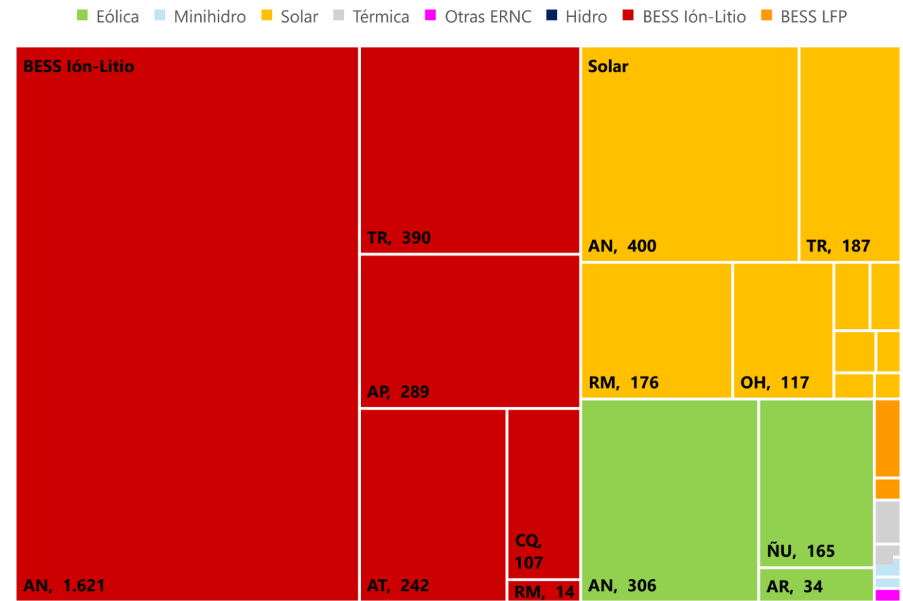
Capacidad (MW) de centrales y sistemas de almacenamiento en pruebas, según tecnología y región, al 31 de agosto de 2026
