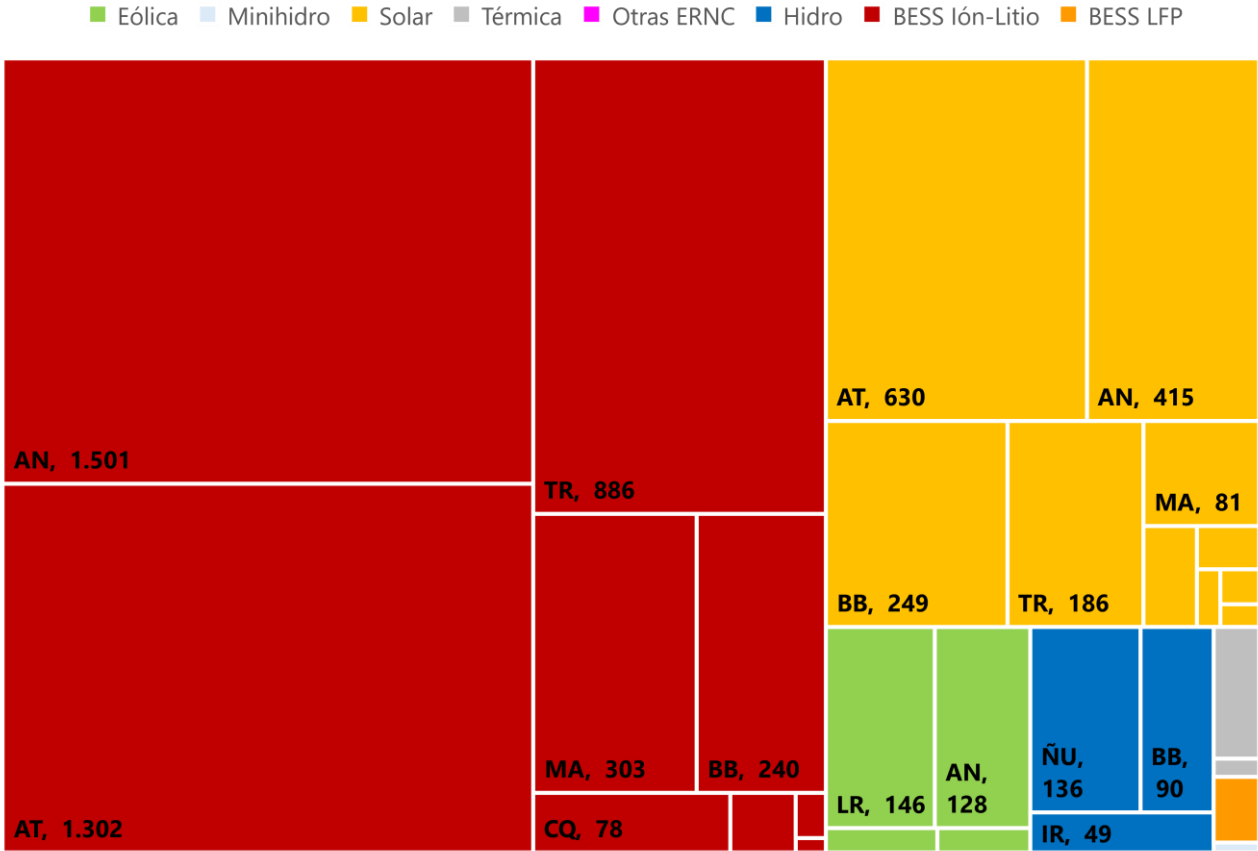
Capacidad (MW) de centrales y sistemas de almacenamiento en construcción, según tecnología y región, al 31 de agosto de 2026
